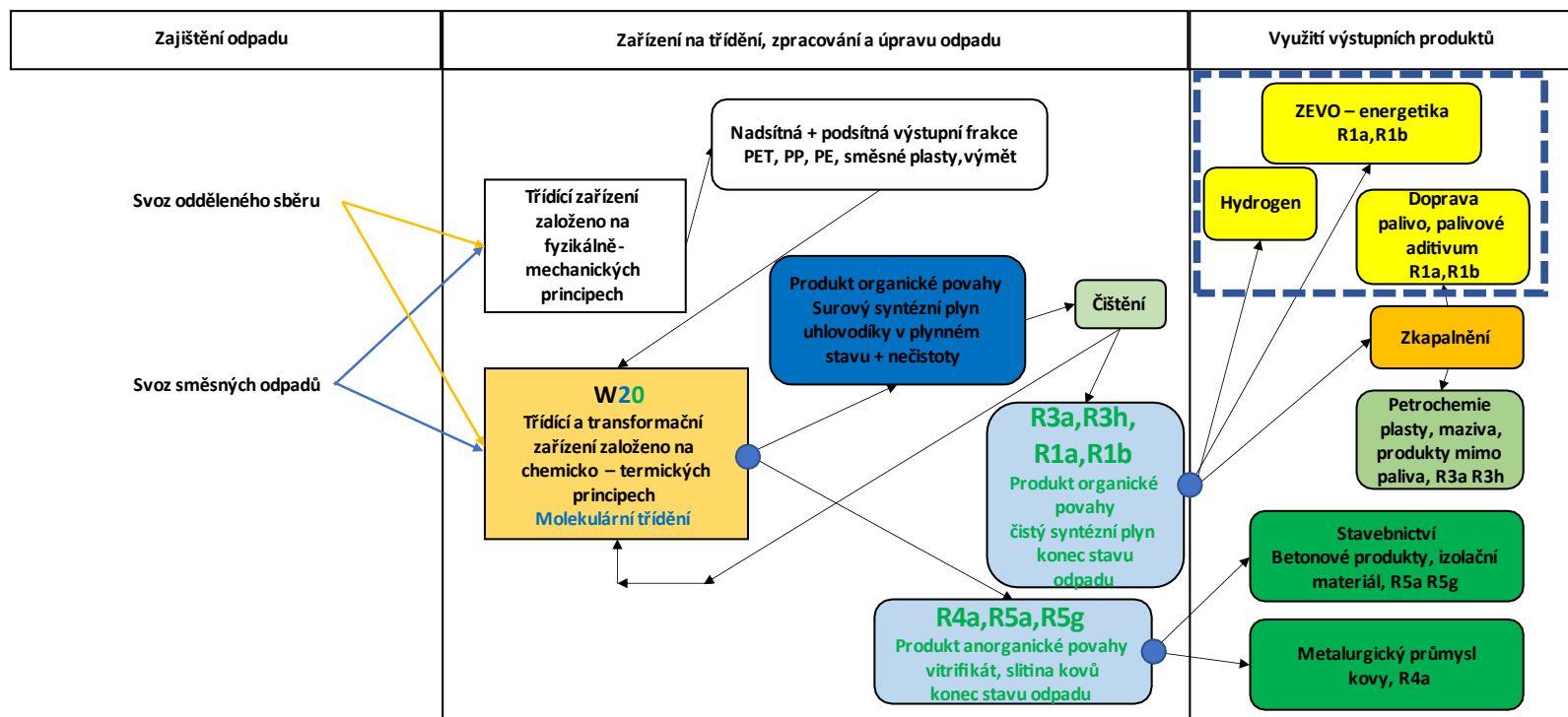
Obr. Diagram chemického procesu zpracování vstupních surovin nebo odpadů na bázi technologie plazmového zplyňování W20 s alternativami využití výstupních produktů
